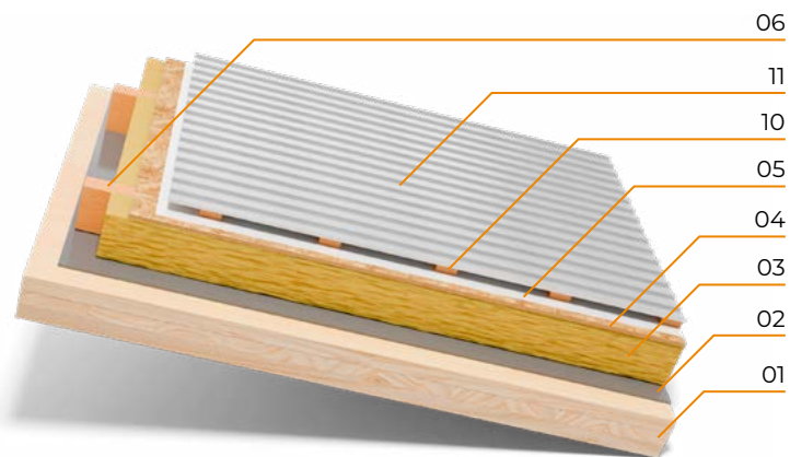
Cubierta ventilada, aislamiento exterior y CLT visto.
