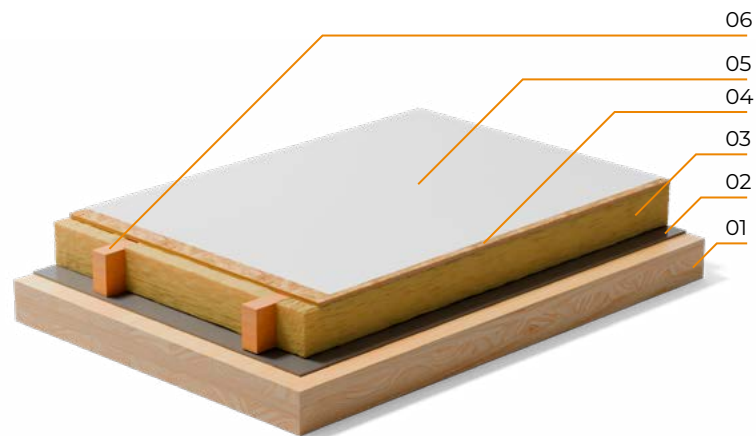
Aislación exterior y CLT visto
