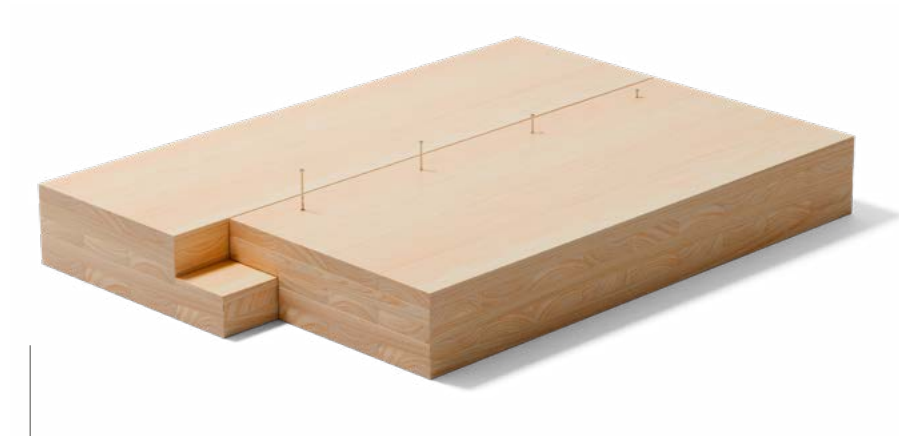
Unión a media madera
