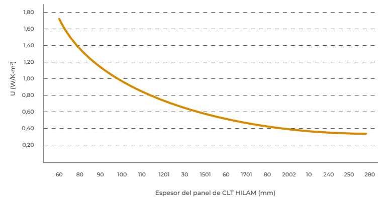
Transmitancia Térmica (U) para elementos de CLT según espesor
