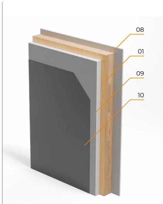
EIFS en el exterior y yeso cartón adherido en el interior
