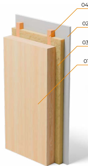
CLT visto y revestimiento con cámara técnica.
