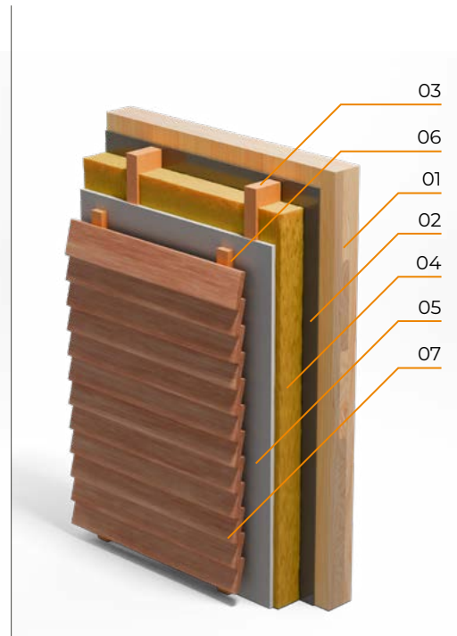
Fachada ventilada y CLT a la vista en el interior
