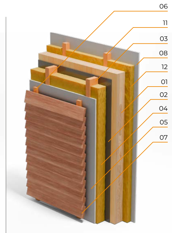
Fachada ventilada y cámara técnica en el interior
