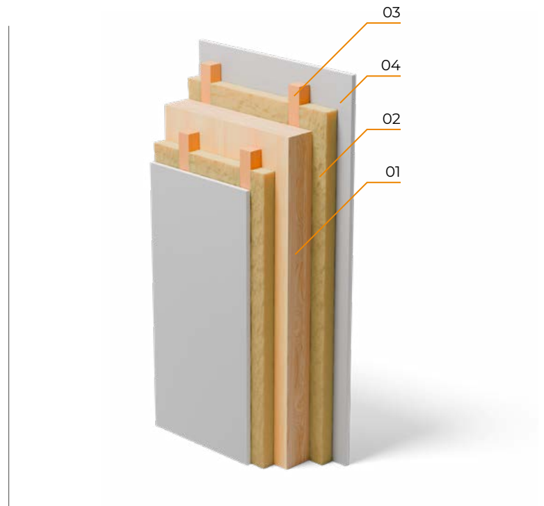
Panel simple de CLT revestido por ambas caras con cámara técnica
