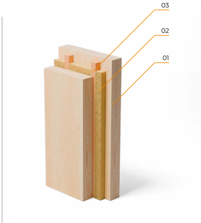
Doble panel de CLT visto
