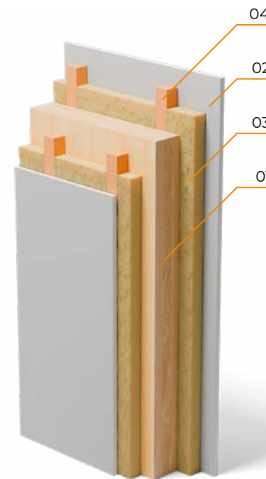
Doble cámara técnica.
