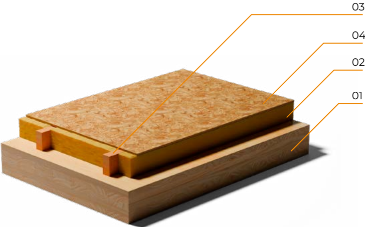
Losa de techo con CLT visto
