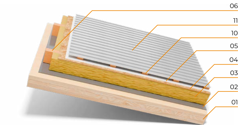
Cubierta ventilada, aislación exterior y CLT visto.
