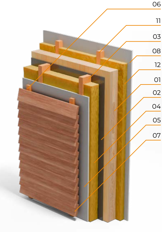
Fachada ventilada y cámara técnica en el interior
