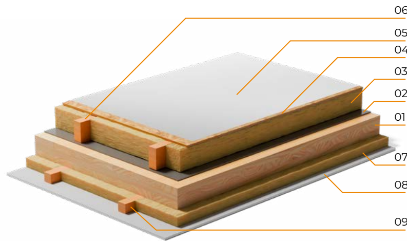
Aislación interior y exterior
