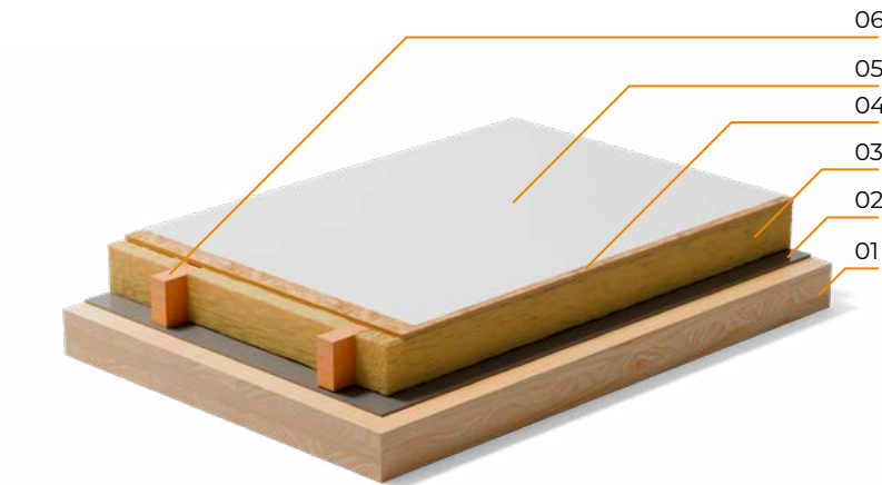
Aislación exterior y CLT visto
