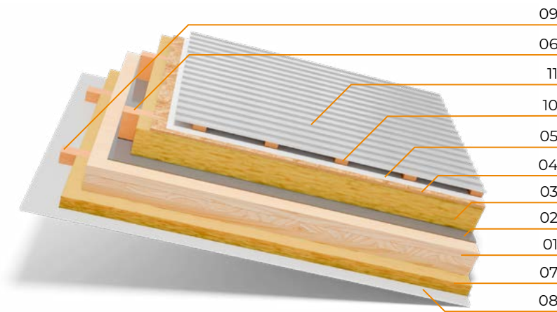
Cubierta ventilada, aislación interior y exterior
