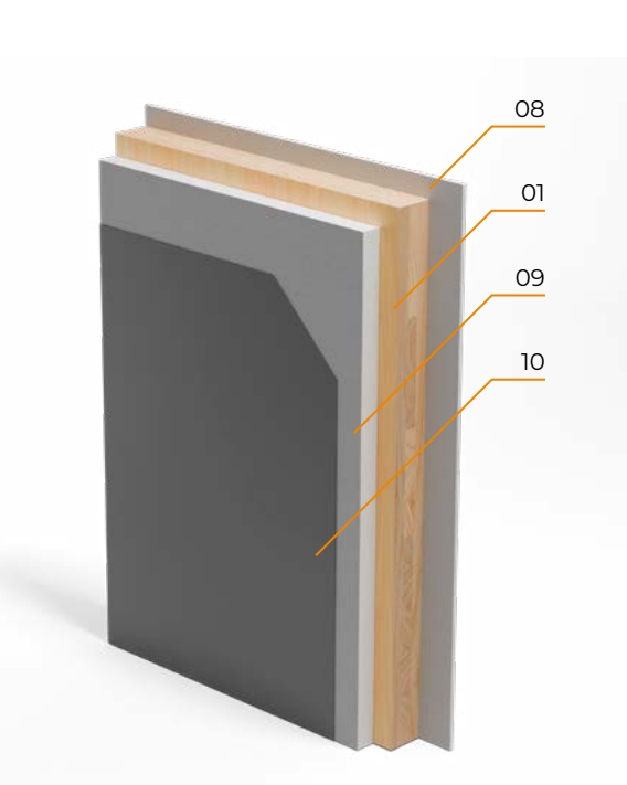
EIFS en el exterior y yeso cartón adherido en el interior
