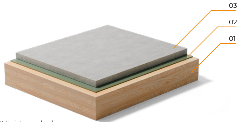
CLT visto y sobrelosa de hormigón
