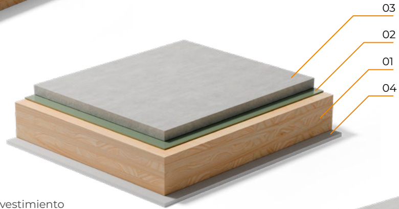
Revestimiento adherido al CLT y sobrelosa de hormigón
