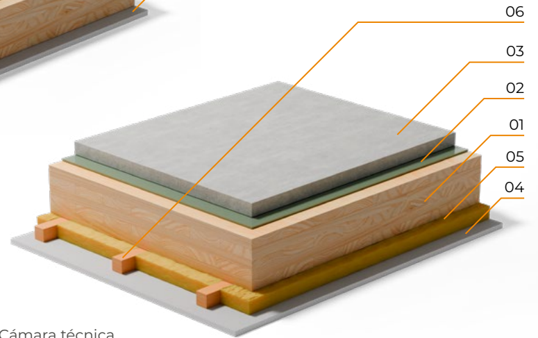
Cámara técnica y sobrelosa de hormigón
